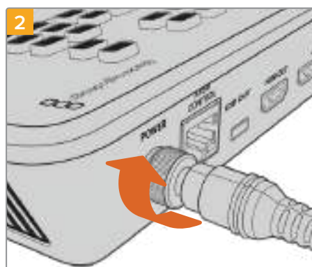
2 コネクタをきつく締めて、ATEM Miniにしっかり固定。
