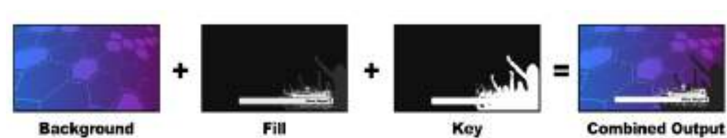
Совмещение фона, заполняющего и вырезающего сигналов при линейном кеинге
